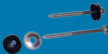
Parafuso com Arruela e Anel de Vedação
